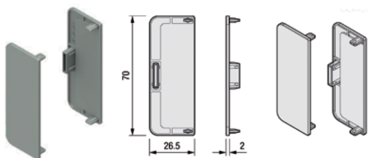
Gola C eindkappen
