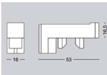
plafondbevestiging muurbevestiging
