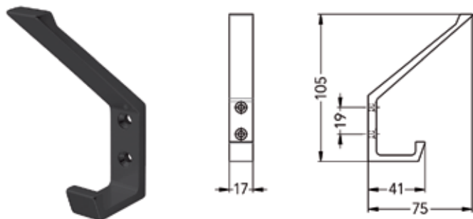
Jashaak type 138 - met haak voor hoed
